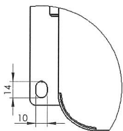
DETAIL A SCALA 1 : 3
