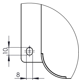
DETAIL C SCALA 1 : 3
